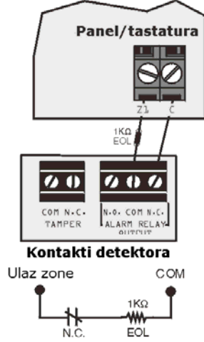
N.C., sa EOL otpornikom, sa prepoznavanjem tampera i prekidom ožičenja (UL/ULC)
