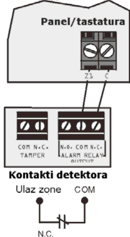
N.C. kontakti, bez EOL otpornika
